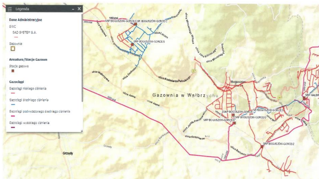
Rysunek 6. Mapa poglądowa dystrybucyjnej sieci gazowej na terenie Gminy Boguszów-Gorce.
