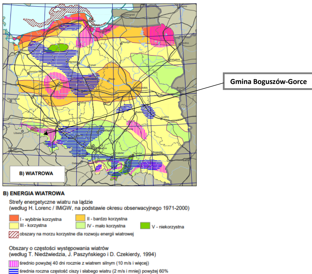
Rysunek 7. Strefy energetyczne wiatru na lądzie (według H. Lorenc/IMI GW, na podstawie okresu obserwacyjnego 1971-2000)
